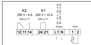
Abb. 3: Anschlusssschema Fig. 3: Connection diagram Fig. 3: Schema de connexion Abb. 3: Aansluitschema Bild 3: Anslutningsschema Fig. 3: Schema d'alimentazione Imagen 3: Esquema de conexión 図 3: 結線図
